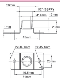
Platine de montage pour veines d'air avec filetage male 1/2". Compatible avec le refroidisseur avec écrou mobile 1/2". Non compatible avec série Y0
