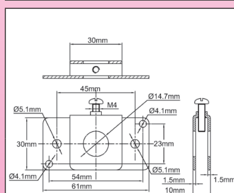
Bride mobile en inox, pour cannes avec bossage de 14.5mm
