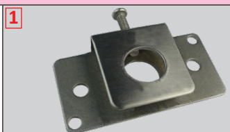
Bride mobile en inox, pour cannes avec bossage de 14.5mm
